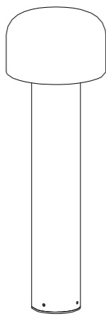
LZ-26712H3-6 D125xH380(mm) LED-6W
