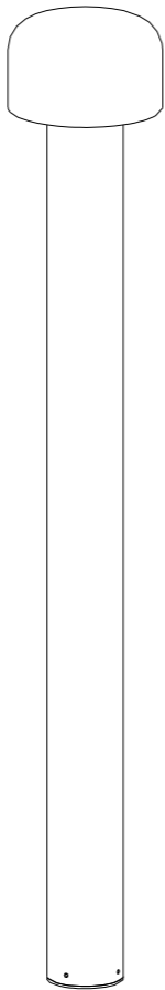
LZ-26712H8-6 D125xH800(mm) LED-6W
